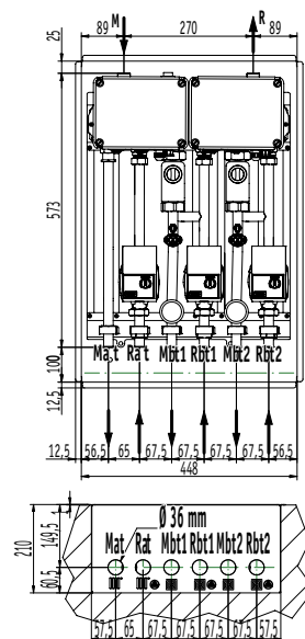
Module partage + (1 zone HT + 2 zones BT)
